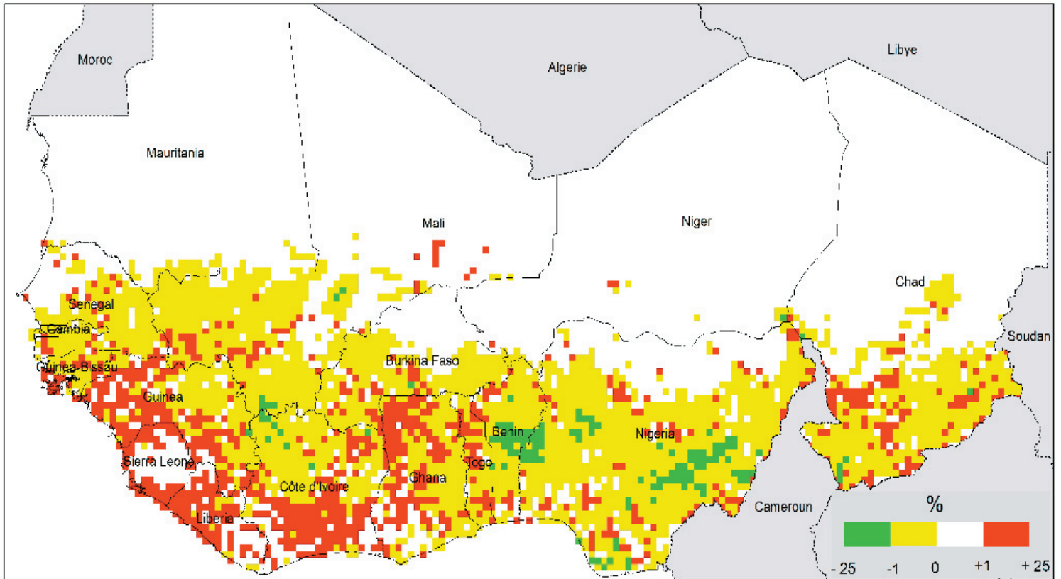
Figure 3 : Comparaison des foyers de feux actifs de la saison 2010/2011 à celle des dix dernières années
