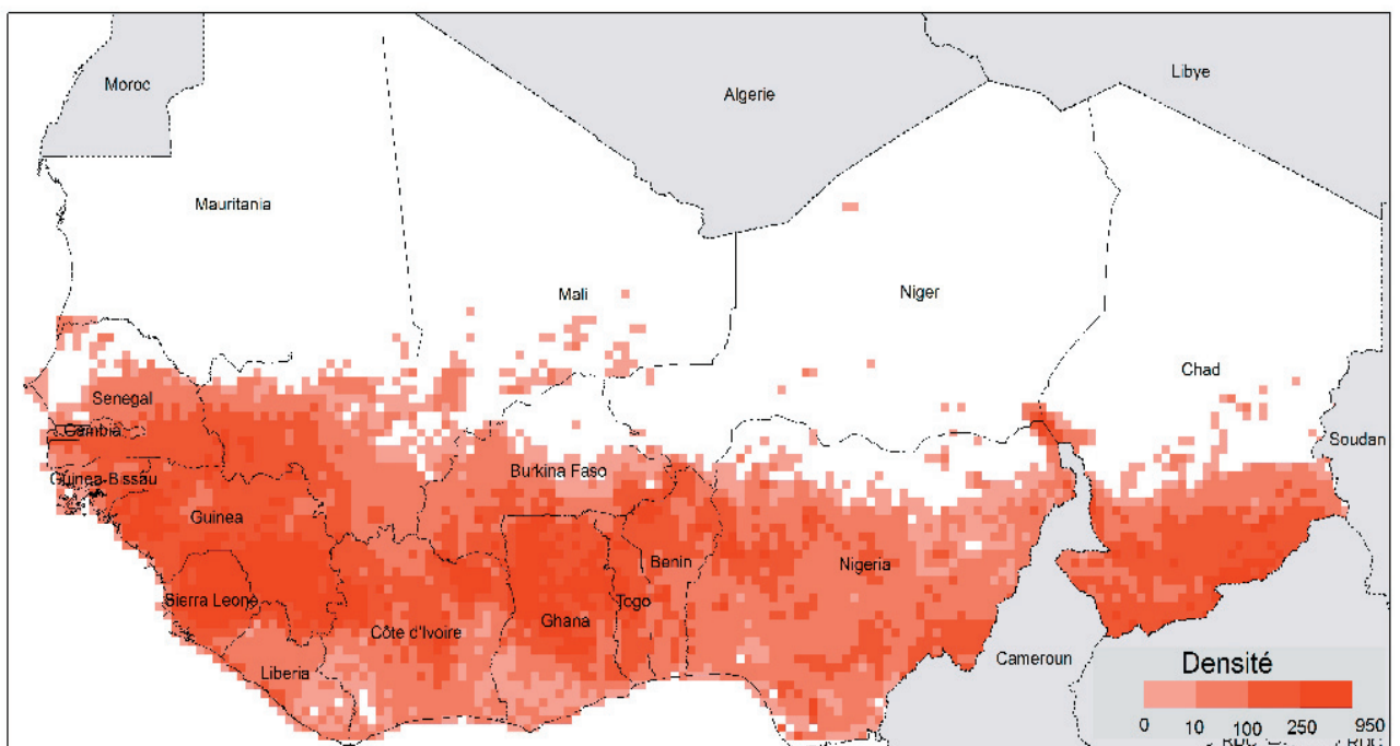
Figure 2 : Densité des foyers de feux actifs en Afrique de l'Ouest et au sahel
