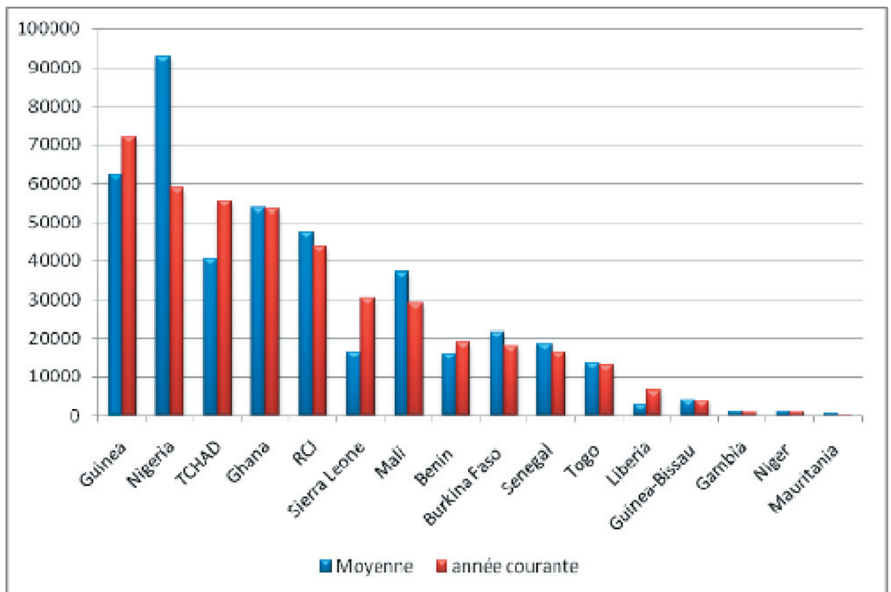
Figure 4 : détection totale de foyers de feux actifs par pays en Afrique de l'Ouest et au Sahel saison 2010/2011
