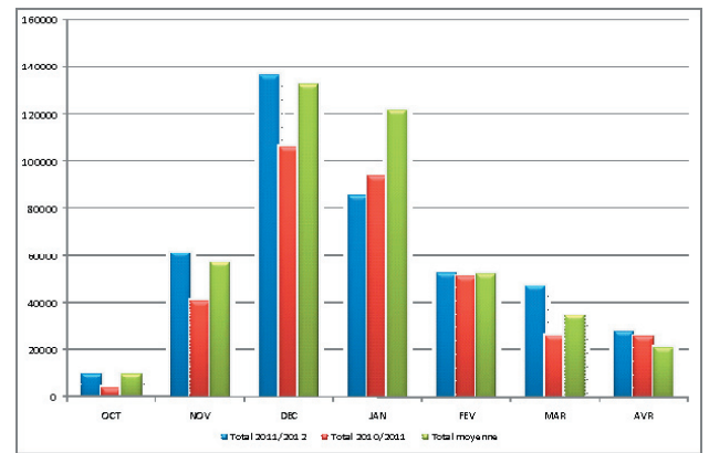
Figure 1: Détections mensuelles de feux actifs en Afrique de l'Ouest et au sahel
