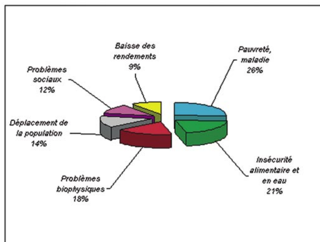
Graphique 1: Conséquences engendrées par la variabilité et les changements climatiques
